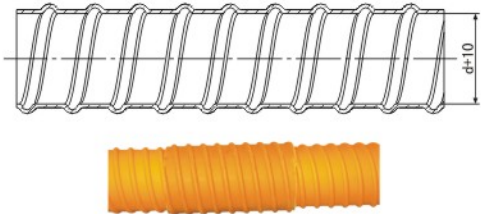
OLG coupler
